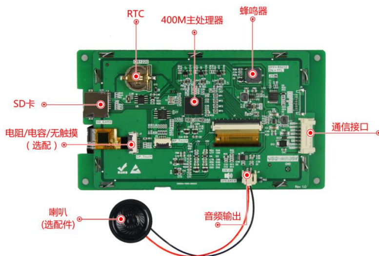
图 1-4 硬件配置图
