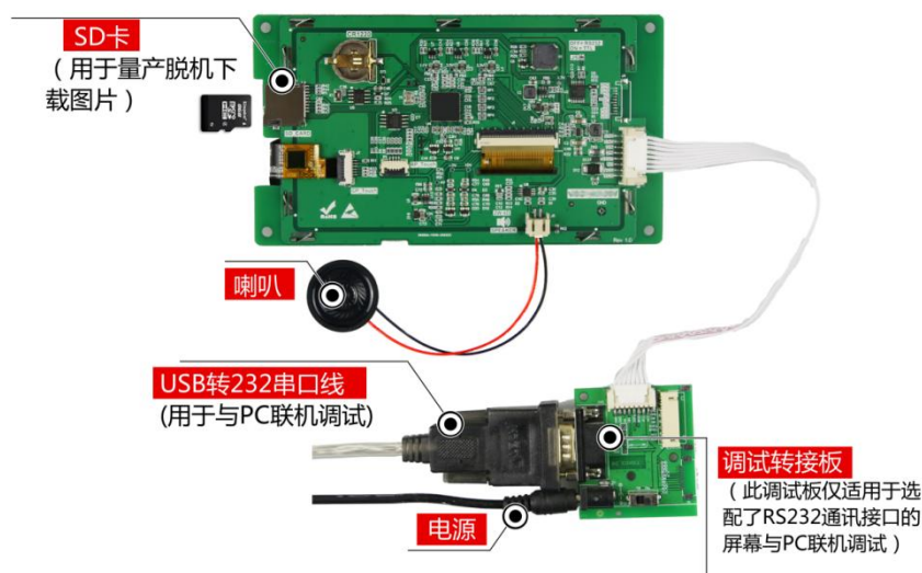
图 1-5 调试工具图
